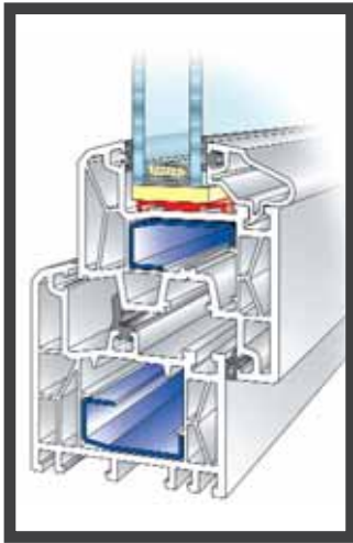
Fenster-System 4000 mit flächenversetztem Flügel 70 mm
