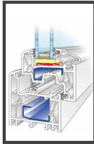
Fenster-System 4000 mit flächenversetztem PROLUX-Flügel 70 mm
