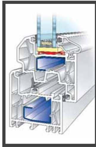
Fenster-System 4000 mit halbflächenversetztem Flügel 77 mm
